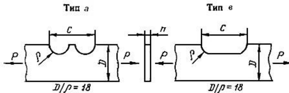
Пластины типов а и в при растяжении
