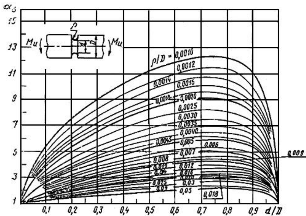
Черт.15. Валы с выточкой при изгибе (черт.14-16)
