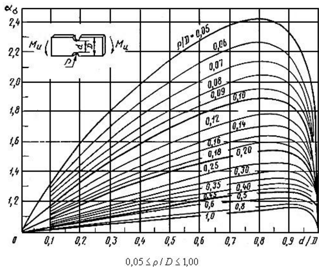
Черт.11. Пластины с двусторонним надрезом при изгибе (черт.9-11)
