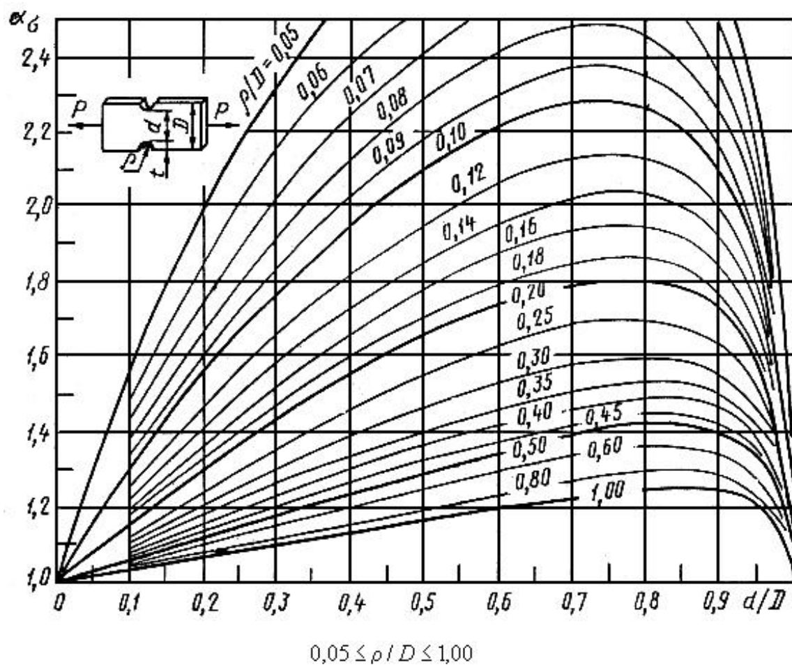
Черт.3. Пластины с двухсторонним надрезом при растяжении (черт.1-3)
