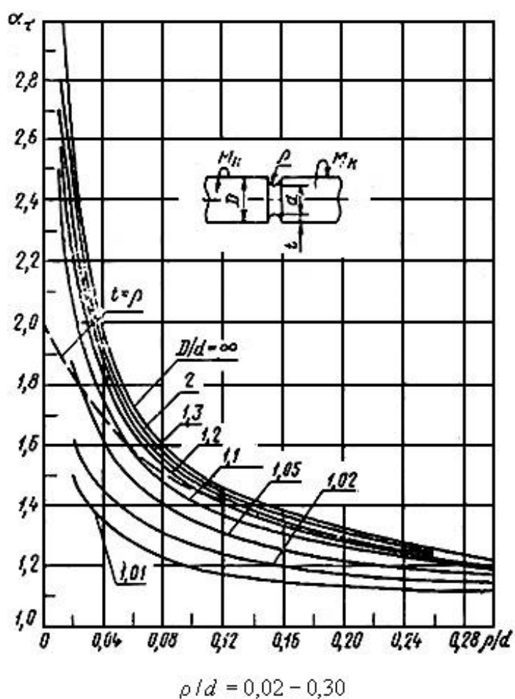
Валы с выточкой при кручении (черт.17-19)
